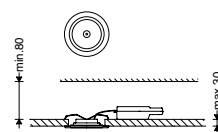
Ø100-105 M219D3ERLED2840-W+ARD4-W
