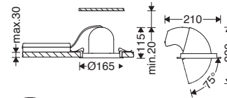
Ø150-155
