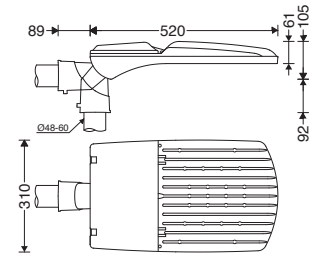
M320XLULED...
