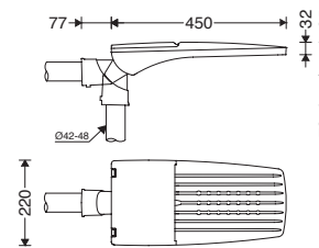
M320MULED5...
