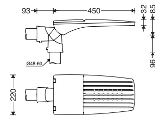
M320MULED6... M320MULED7...
