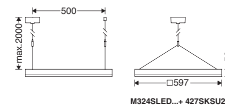
M324SLED...+ 427SKSU2-W
