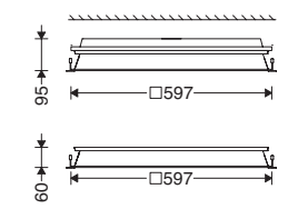
M323SLED...+528SH-W
