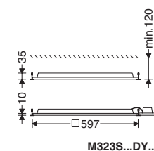
M323S...DY...
