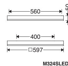
M324SLED...
