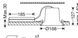
M587...Q15LED... □150 +3
