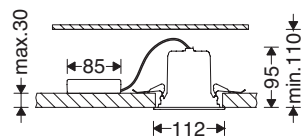
M587EMQ10LED...
